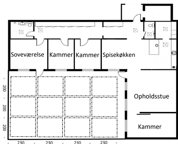
Modulnet i stor bolig type 114 kvm
