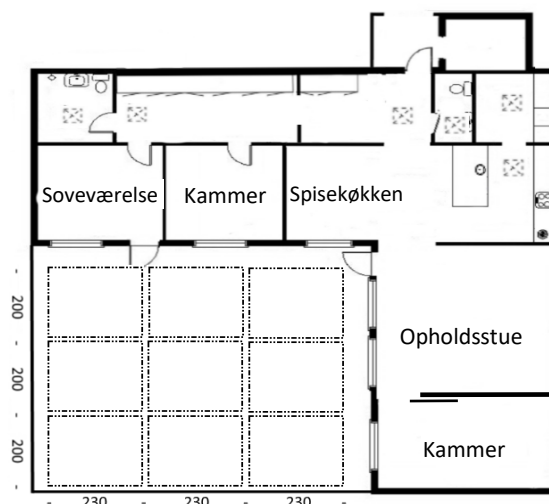
Modulnet i lille bolig type 102 kvm
